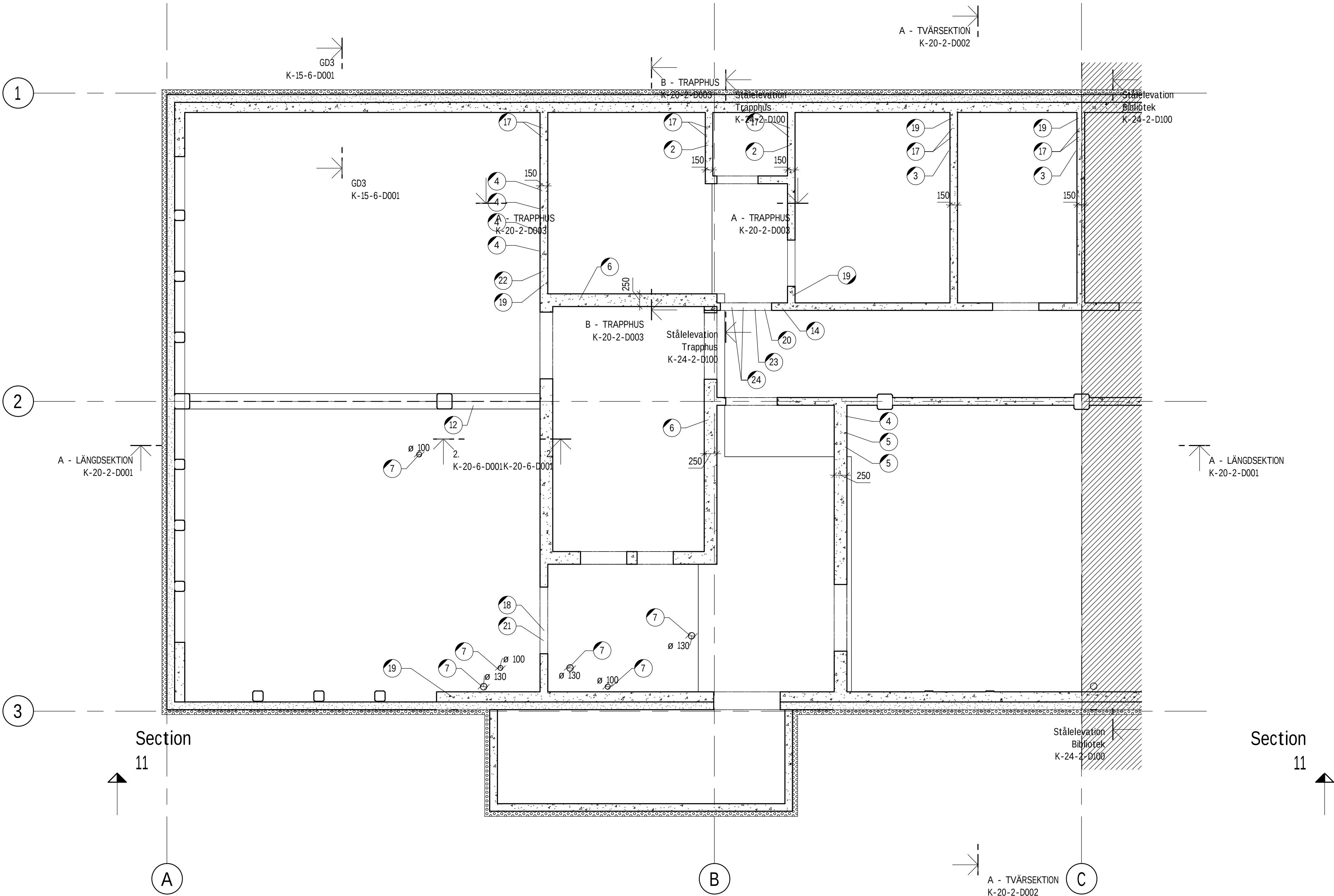
KÄLLARPLAN - Del 1 1 : 50
